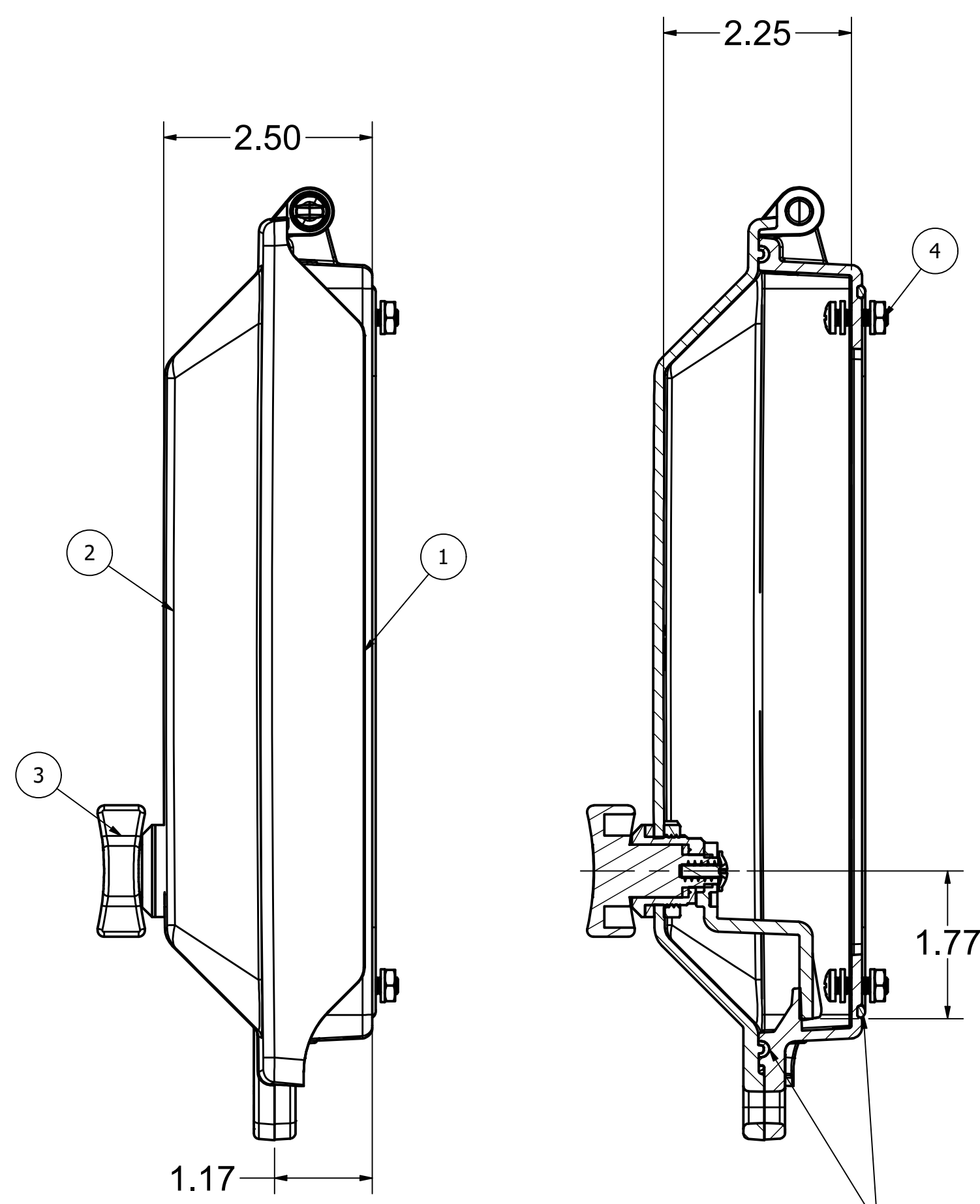
SECTION A-A
